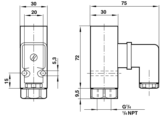
Desenho Dimensional 02
